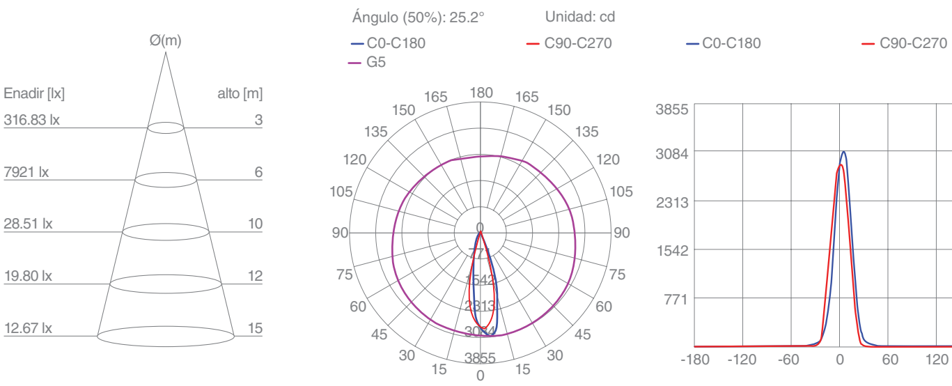
AR111 PRO 11W 24°
