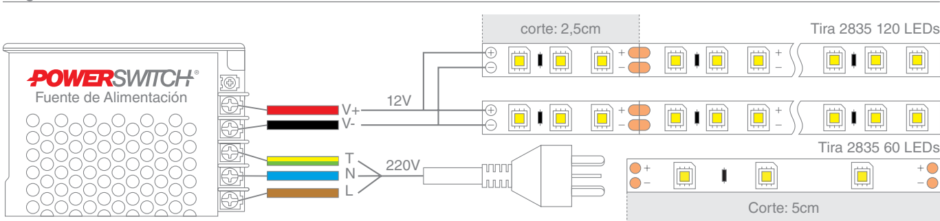
Diagrama de conexión
