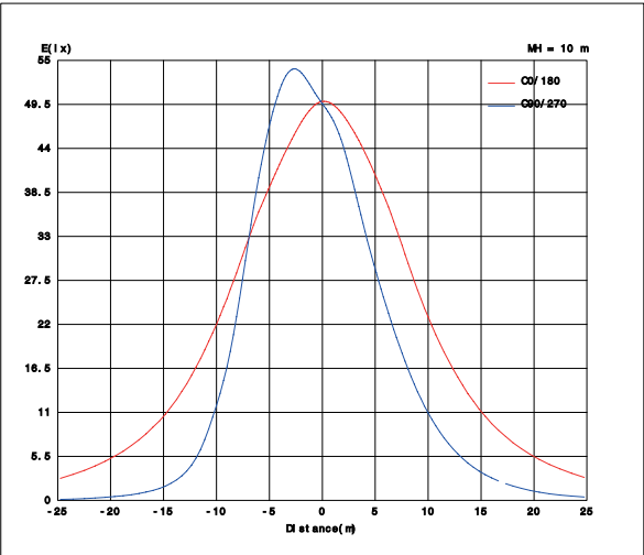
CURVA DE ILUMINANCIA PLANA
