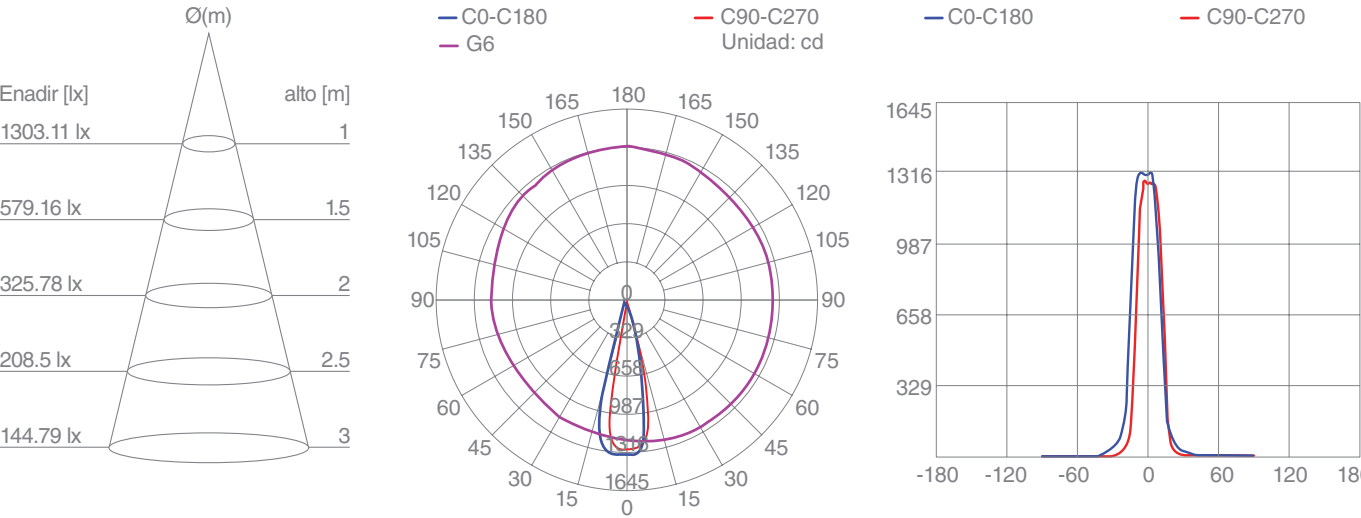
MR16 PRO 5W 24°
